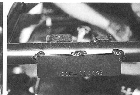
フレーム号機打刻位置 (フレーム左フロント部)
